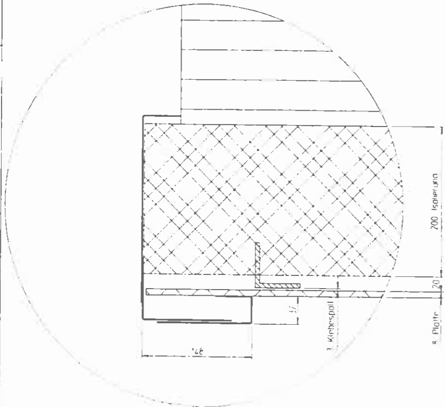
Detail 1 Maßstab 1:2.5
