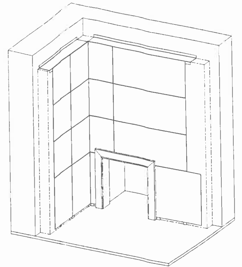
Detail 2 Maßstab 1:2.5
