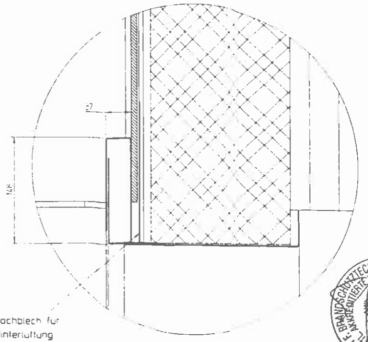
Detail 2 Maßstab 1:2.5
